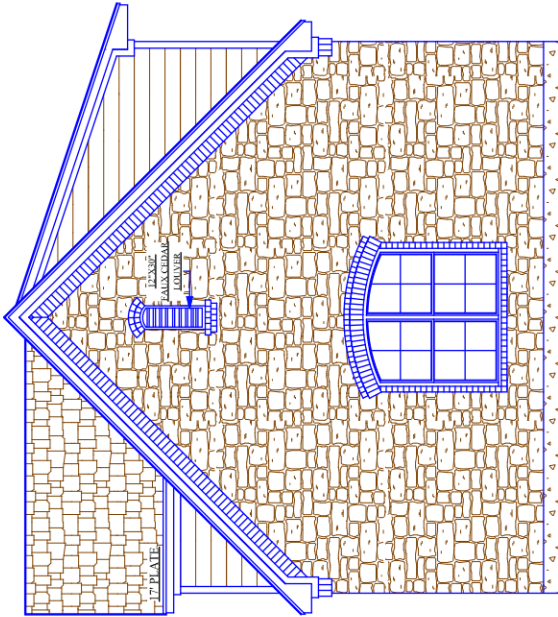
RIGHT ELEVATION
